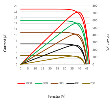
Curvas de corrente-tensão e potência-tensão (700W)
